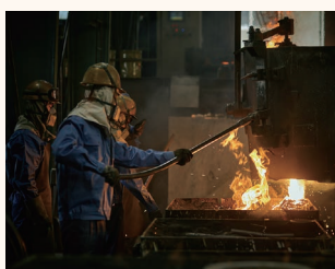
材料を溶解する温度は約1600℃。材料づくりから仕上げまでの一貫生産。
